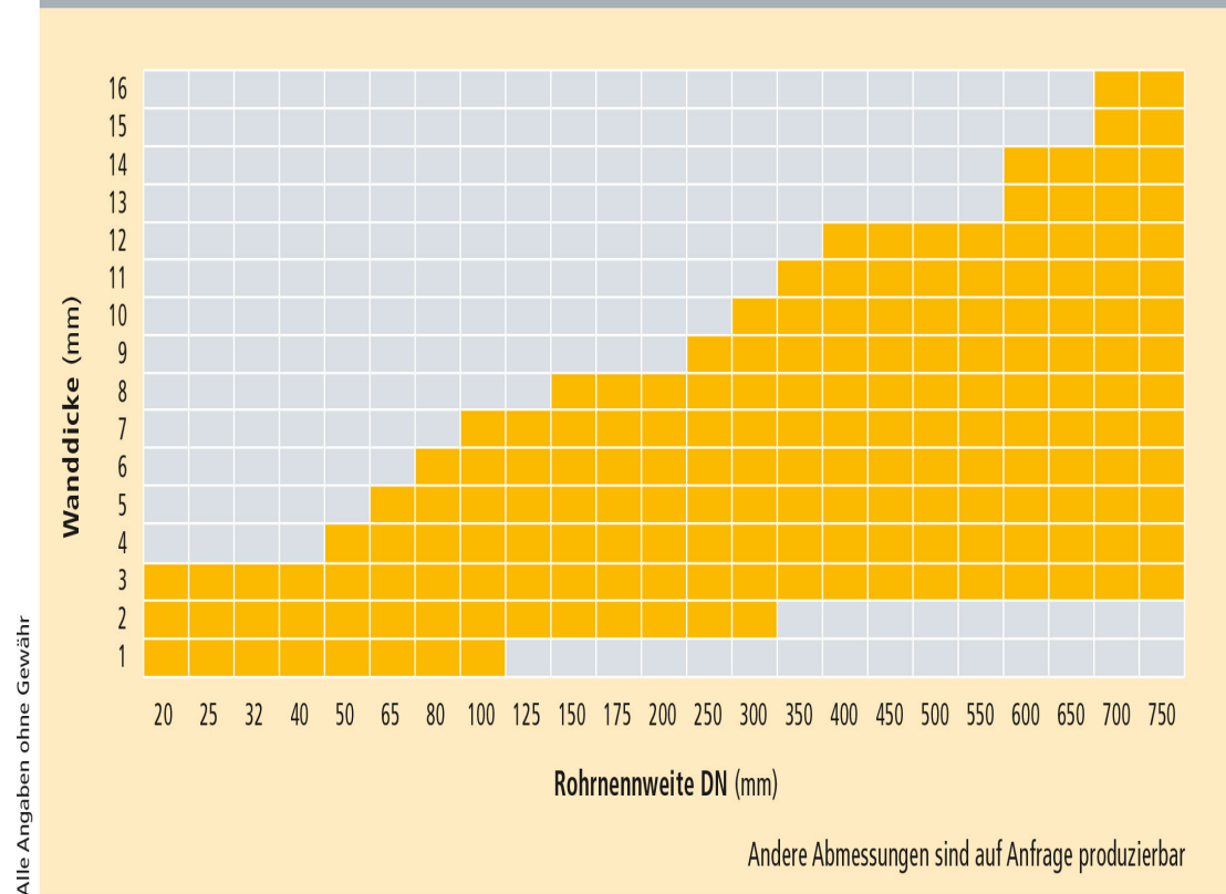
Abb. 1.1.2_1: Mögliches Abmessungsspektrum für Bandrohre
